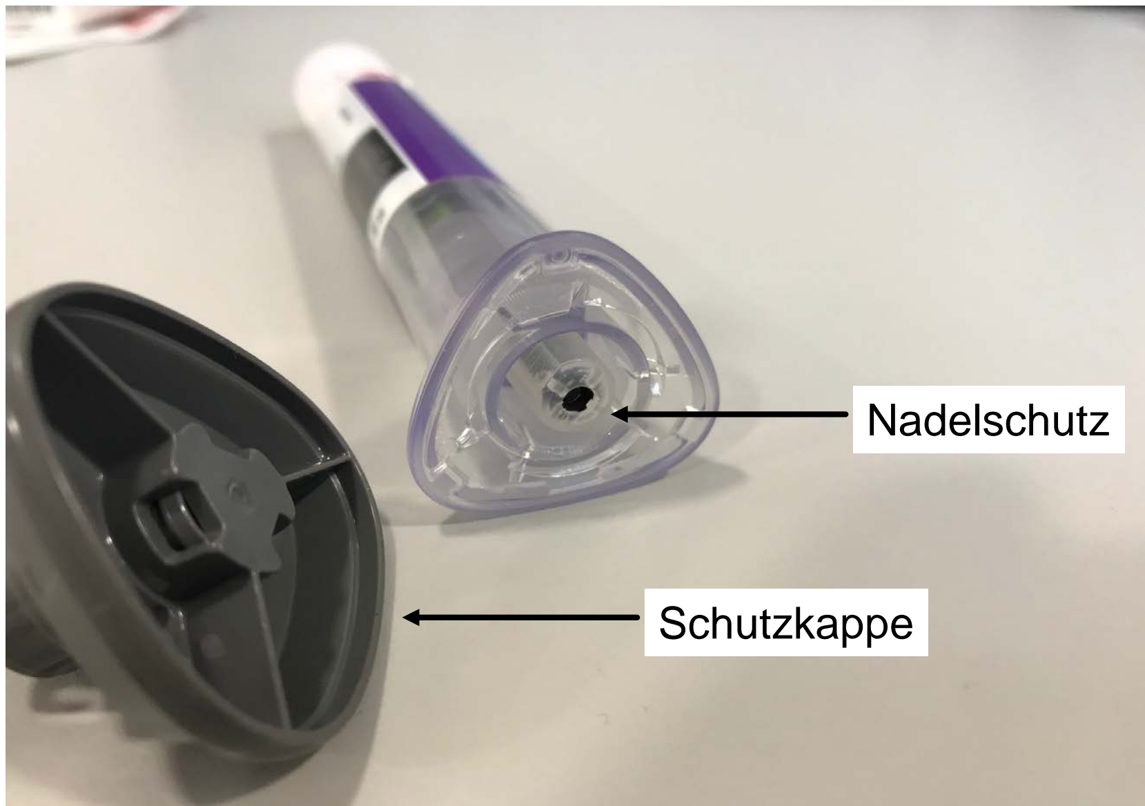
Abbildung: Ansicht eines defekten Trulicity® Fertigpens der Charge D187396 mit abgezogener grauer Schutzkappe (links im Bild). Im Pengehäuse befindet sich noch der Nadelschutz (Bildmitte), der beim Abziehen der Schutzkappe hätte mit entfernt werden sollen. Foto: Quelle AMK
